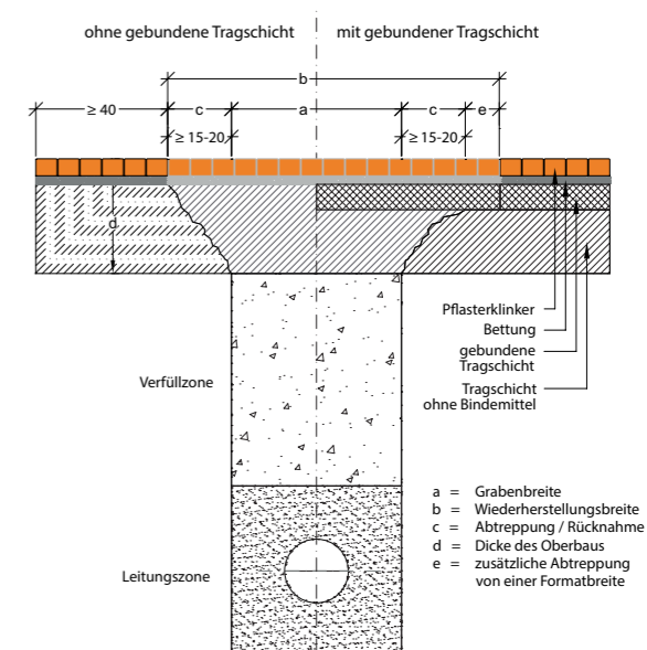
Abb. 6-2: Abtreppung bei Pflasterdecken und Plattenbelägen gemäß den ZTV A-StB
